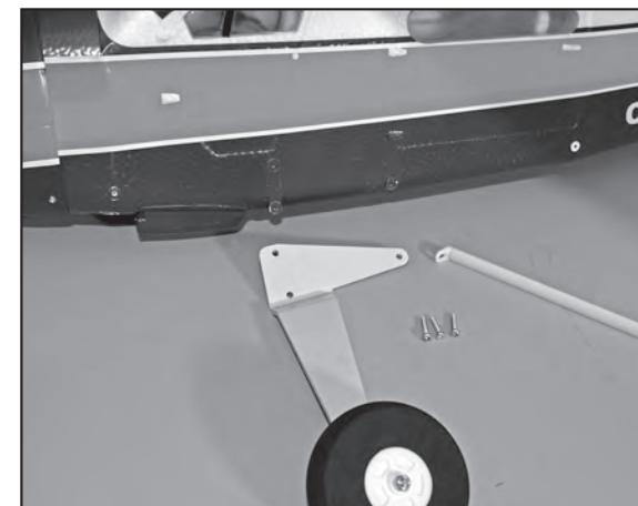
Schrauben der Fahrwerke lösen, Fahrwerke abnehmen.
