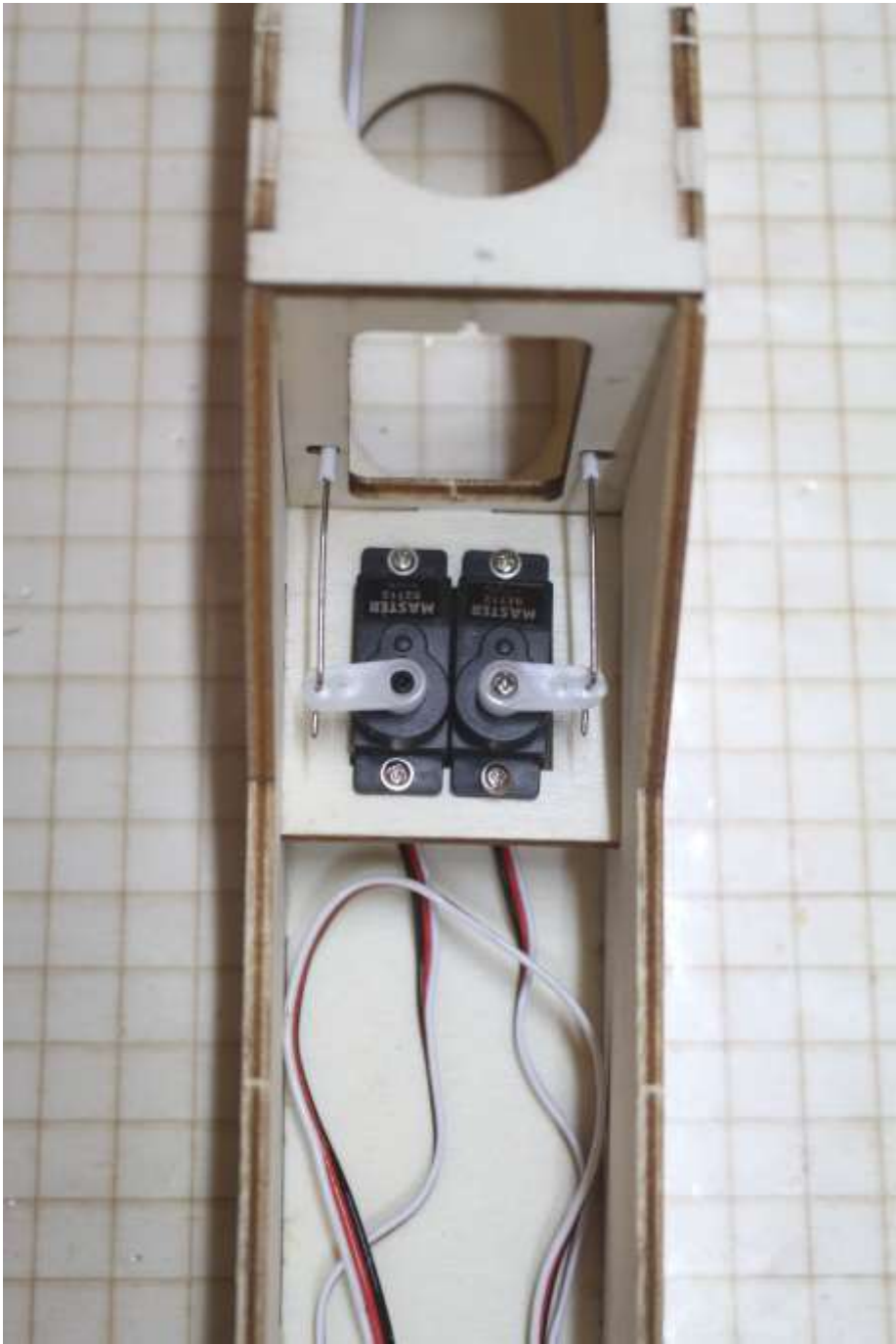
Servos mittels Sender/Empfänger in Neutralstellung bringen Anlenkungsdraht mit Servohebel in Bowdenzurohr einfädeln Servohebel auf Servo aufsetzen und verschrauben
